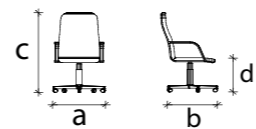
PEG EXW 1100 a: 595 mm b: 638 mm c: 1130-1240 mm d: 420-530 mm
